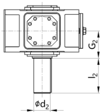
P4SV 实心轴
