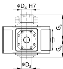
V2DV 带锁紧盘的空心轴
