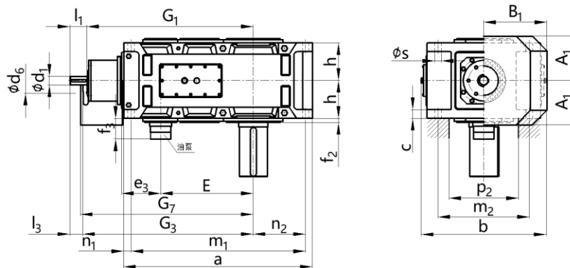
V3HV 空心轴
