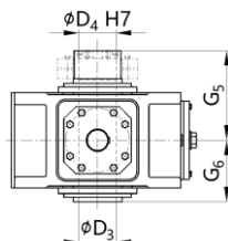
V3DV 带锁紧盘的空心轴
