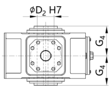
V3HV 空心轴
