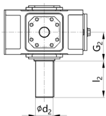
V2SV 实心轴
