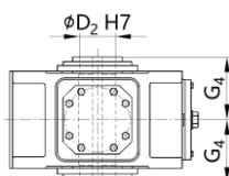
P4HV 空心轴
