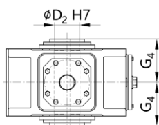
V2HV 空心轴
