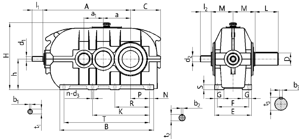
DCY 减速机外形尺寸表
