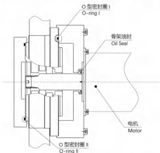
BXJ-110E及以上型号密封示意图 The seal diagram of BXJ-110E and the bigger
