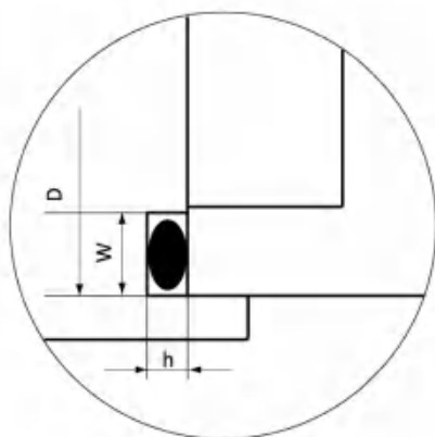
E系列 O 型圈 II 局部放大图
