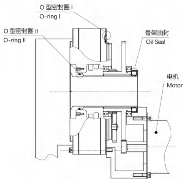
BXJ-C系列密封示意图 The seal diagram of BXJ-C
