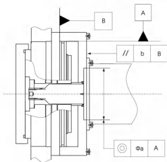
BXJ-80E及其以下型号装配精度示意图 The assembly diagram of BXJ-80E and the smaller
