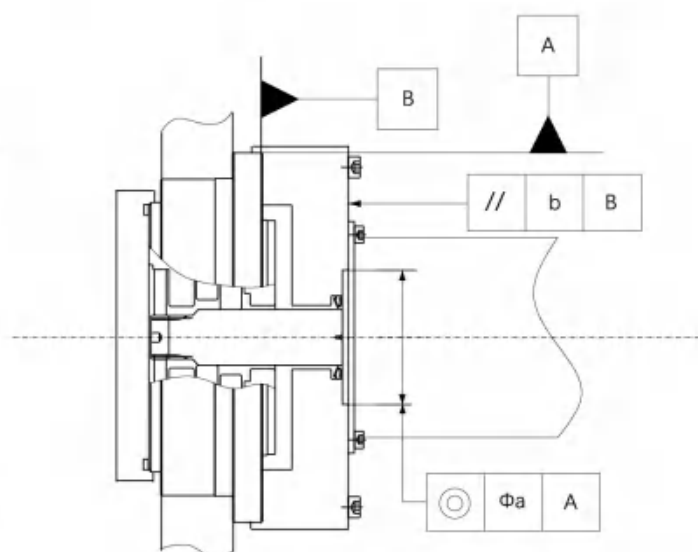
BXJ-110E及其以上型号装配精度示意图 The assembly diagram of BXJ-110E and the bigger
