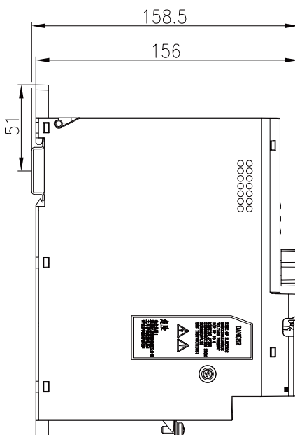
M1 (0.75kw~5.5KW) 外形尺寸图, 单位为mm
