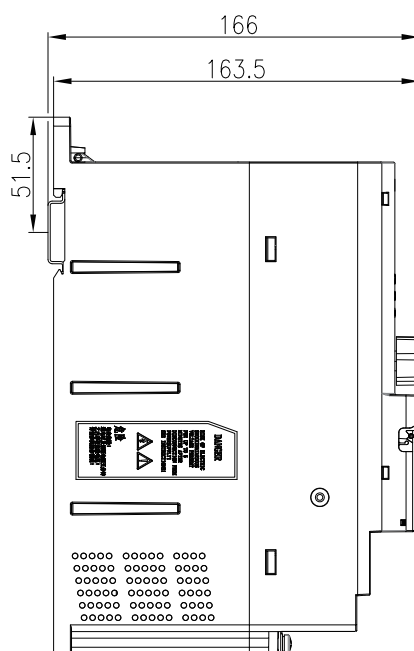
M2 (5.5kW) 外形尺寸图, 单位为mm
